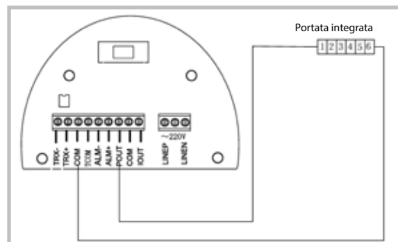
Fig. 6c Connessione del contatore elettronico (uscita passiva necessita 24 Vcc dal PLC) ed eventuale resistenza da 1 o 2 KOhm, se non prevista nell'acquisitore
