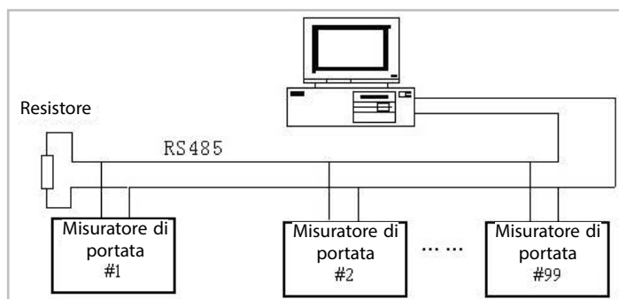
Fig. 1 Struttura della rete del misuratore di portata elettromagnetico
