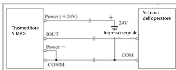
Fig. 11 Misuratore S-MAG, tre connessioni (alimentazione e uscita in corrente non sono isolate)
