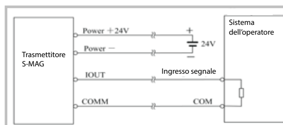
Fig. 12 Misuratore S-MAG, quattro connessioni (alimentazione e uscita in corrente sono isolate)
