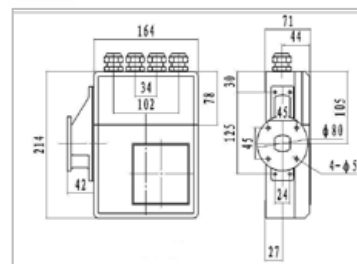
Dimensioni vano elettronica versione separata
