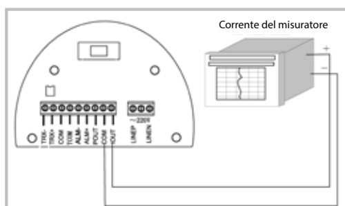
Fig. 6a Circuito corrente in uscita attiva (non necessita alimentazione 24 Vcc)
