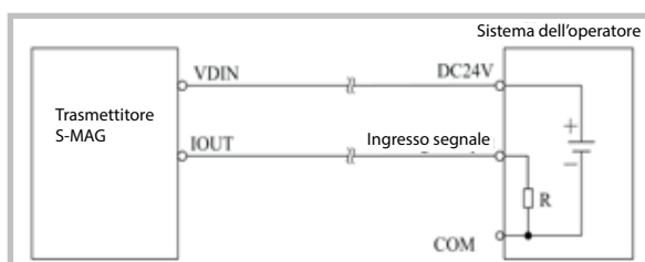
Fig. 10 Misuratore S-MAG, due connessioni
