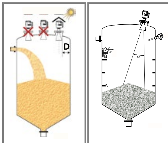
Riempimento laterale
