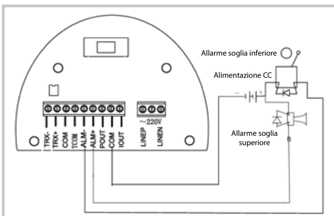
Fig. 6d Connessione dell'uscita di allarme
