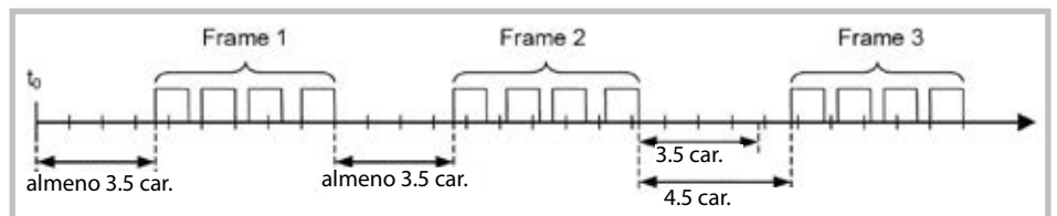
Fig. 4 Intervallo del frame MODBUS
