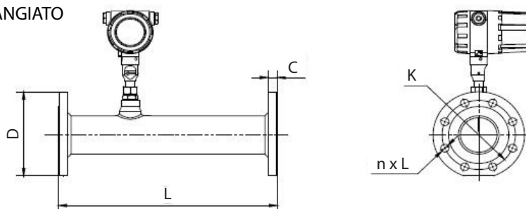
SENSORE FLANGIATO
