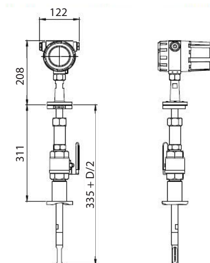
SENSORE A INSERZIONE CON GIUNTO A COMPRESIONE
