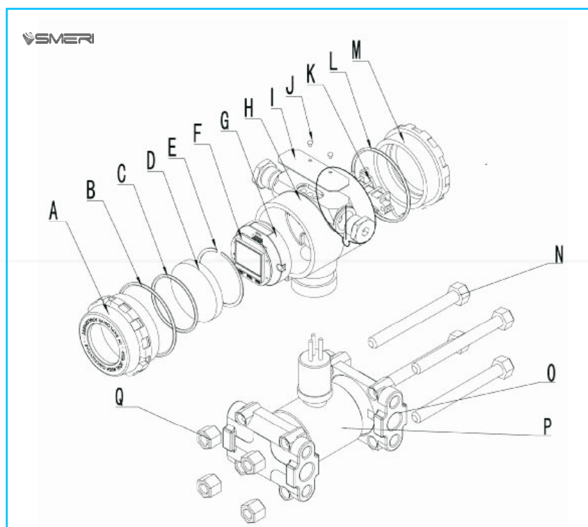
Elementi del trasmettitore di pressione
