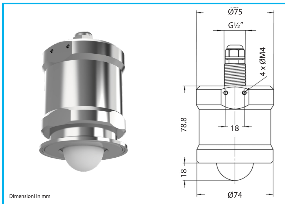
MINIRADAR S-810-L in acciaio inox 304, connessione flangiata o filettata
