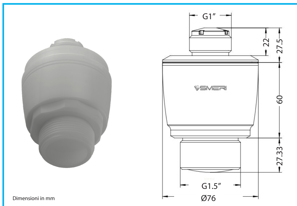
MINIRADAR S-810-EL in PVDF, connessione filettata o flangiata
