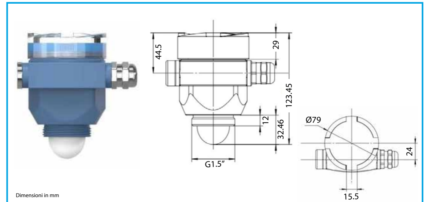
MINIRADAR S-800-RL in PBT+GF con display, attacco filettato 1 1/2" G, configurazione locale mediante tasti operativi o wireless
