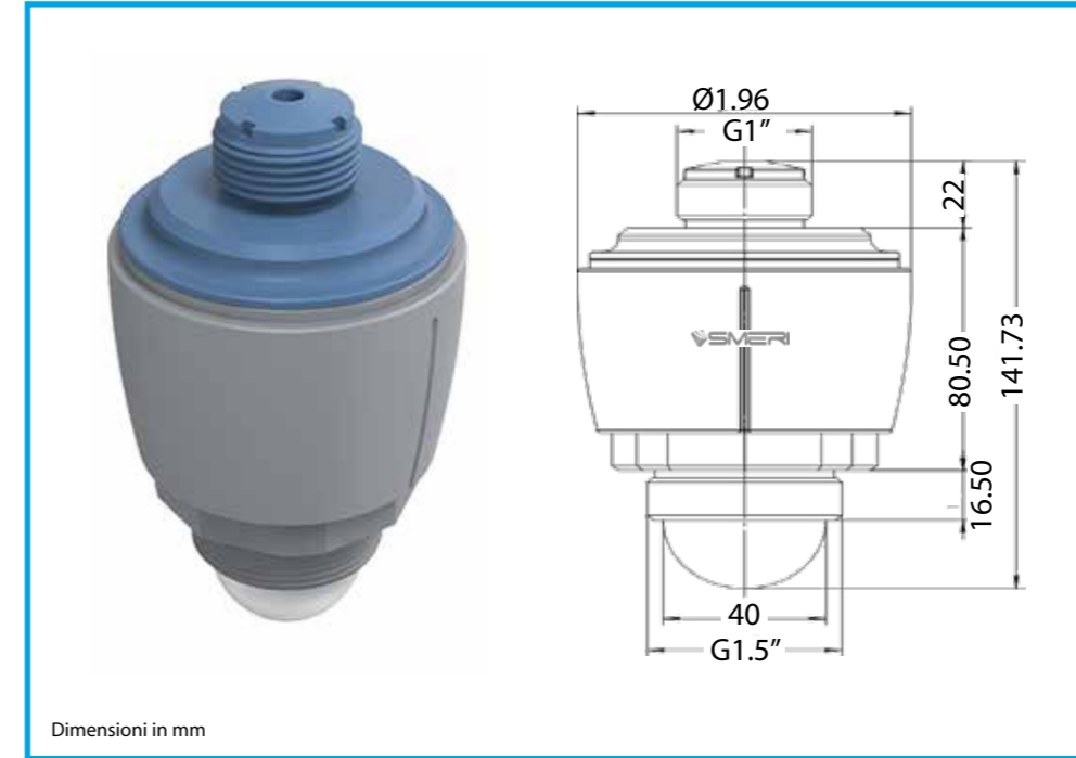
MINIRADAR S-811-L standard plus in GFPP, connessione filettata o flangiata
